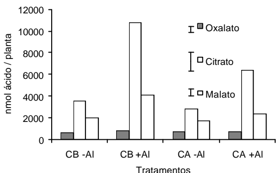
Figura 4. Exudação de ácidos orgânicos pelos cultivares de arroz Comum Branco(CB) e caiapó(CA), na presença (+) ou ausência (-) de Alumínio (Al), por um período de 15 dias de exposição ao elemento. A barra ao lado da legenda indica a DMS para cada ácido, respectivamente.
