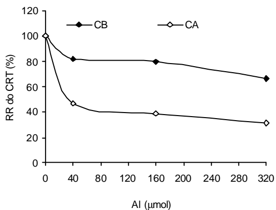
Figura 1. Redução relativa da área (ART) e do comprimento (CRT) radicular total das variedades de arroz de sequeiro Comum Branco (CB) e Caiapó (CA) em período de 4 dias de exposição ao Al.
