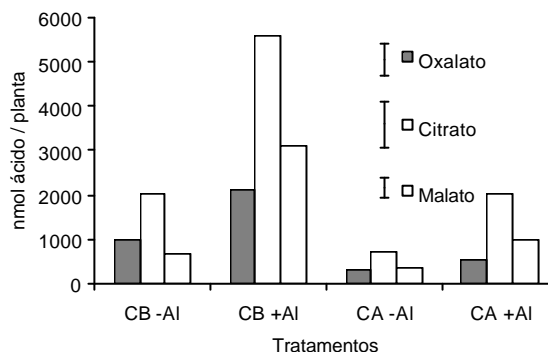
Figura 6. Conteúdo de ácidos orgânicos acumulados nas raízes dos cultivares de arroz Comum Branco (CB) e Caiapó (CA), na presença (+) ou ausência (-) de Alumínio (Al), por um período de 15 dias de exposição ao elemento. A barra ao lado da legenda indica a DMS para cada ácido, respectivamente.
