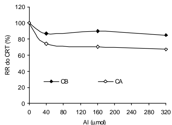
Figura 2. Redução relativa da área (ART) e do comprimento (CRT) radicular total das variedades de arroz de sequeiro Comum Branco (CB) e Caiapó (CA) em período de 15 dias de exposição ao Al.
