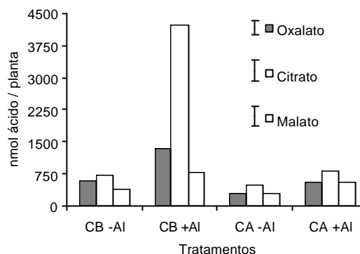
Figura 5. Conteúdo de ácidos orgânicos acumulados nas raízes dos cultivares de arroz Comum Branco (CB) e Caiapó (CA), na presença (+) ou ausência (-) de Alumínio (Al), por um período de 4 dias de exposição ao elemento. A barra ao lado da legenda indica a DMS para cada ácido, respectivamente.
